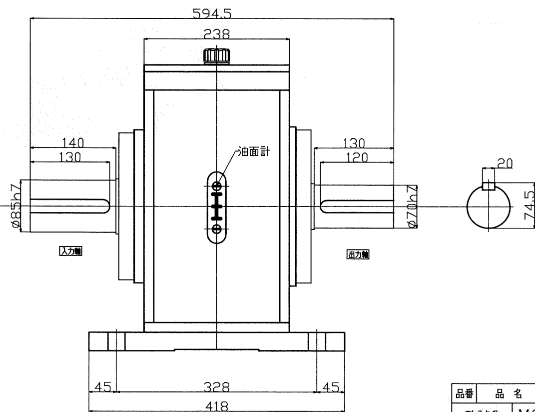
132 kw用2倍增速機
